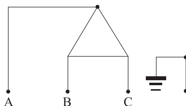
角型接线图
