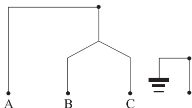
星型接线图
